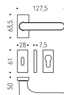
CC 21 RSM-RSMY Wykończenia: C01 - C02 - C03 - C04 - C05 - C06 C07 - C08 - C09 - C10 - C11 - C12
