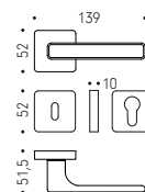
CC 41 R-RY Ø50 Wykończenia: C01 - C02 - C03 - C04 - C05 - C06 C07 - C08 - C09 - C10 - C11 - C12
