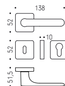
CC 21 R-RY 52x52 Wykończenia: C01 - C02 - C03 - C04 - C05 - C06 C07 - C08 - C09 - C10 - C11 - C12
